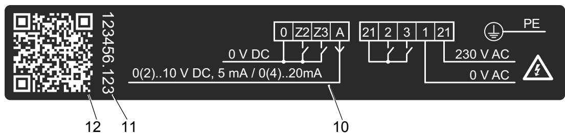
3-2: Anslutningsschema (exempelbild)
