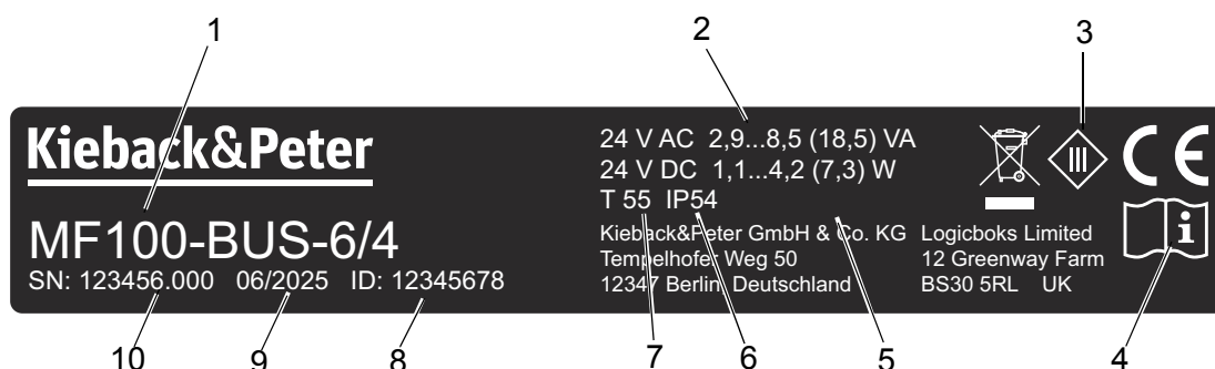
3-1: Ställdonets typskylt (exempelbild)
