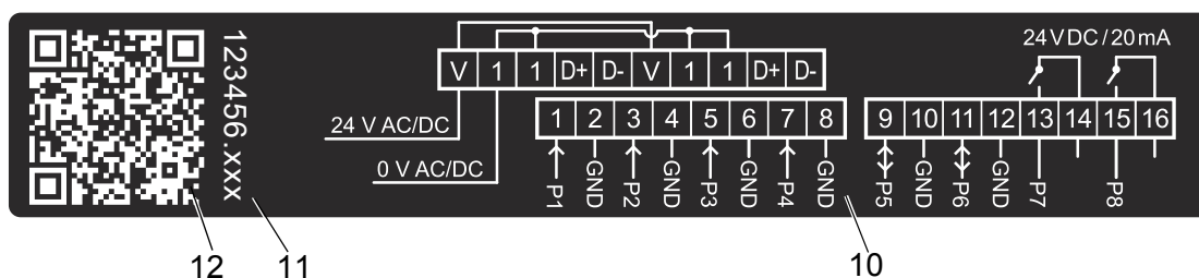
3-2: Anslutningsschema (exempel)
