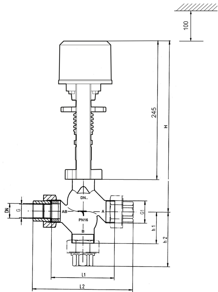
Utförande RB .. -BK (flödesventil) med blindlock på öppning B
